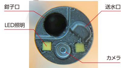
挿入部先端構造
